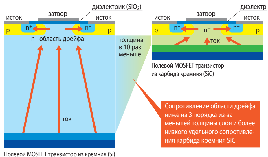
Рис. 2. Упрощенная структура полевого транзистора MOSFET
