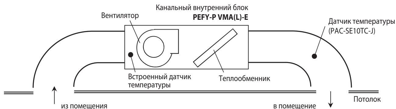
Рис. 1. Расположение датчиков температуры
