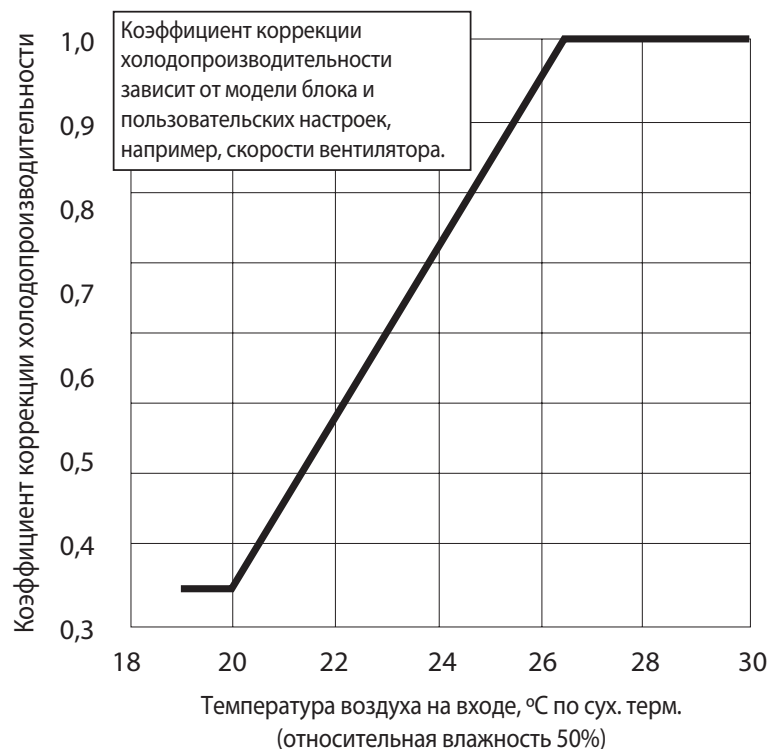
Рис. 2. Коррекция холодопроизводительности
